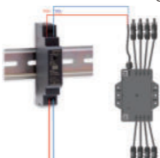
Abb. I: Befestigung der Stromversorgung an der Schiene
