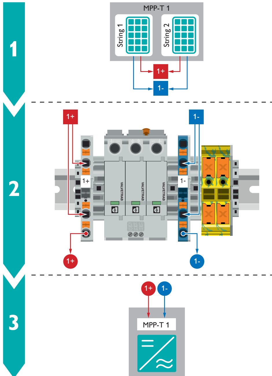
Anschlusszeichnung
