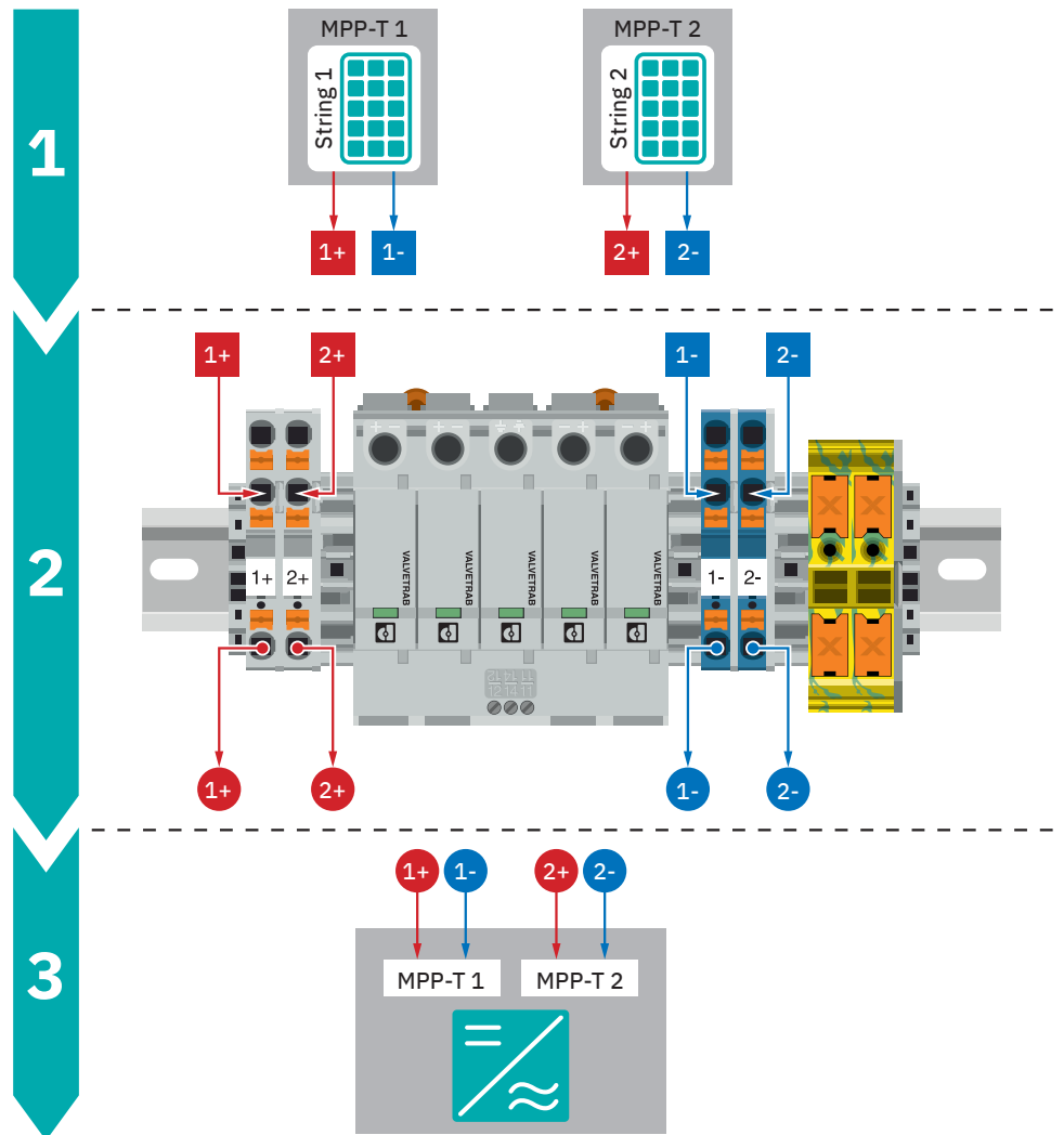
Anschlusszeichnung
