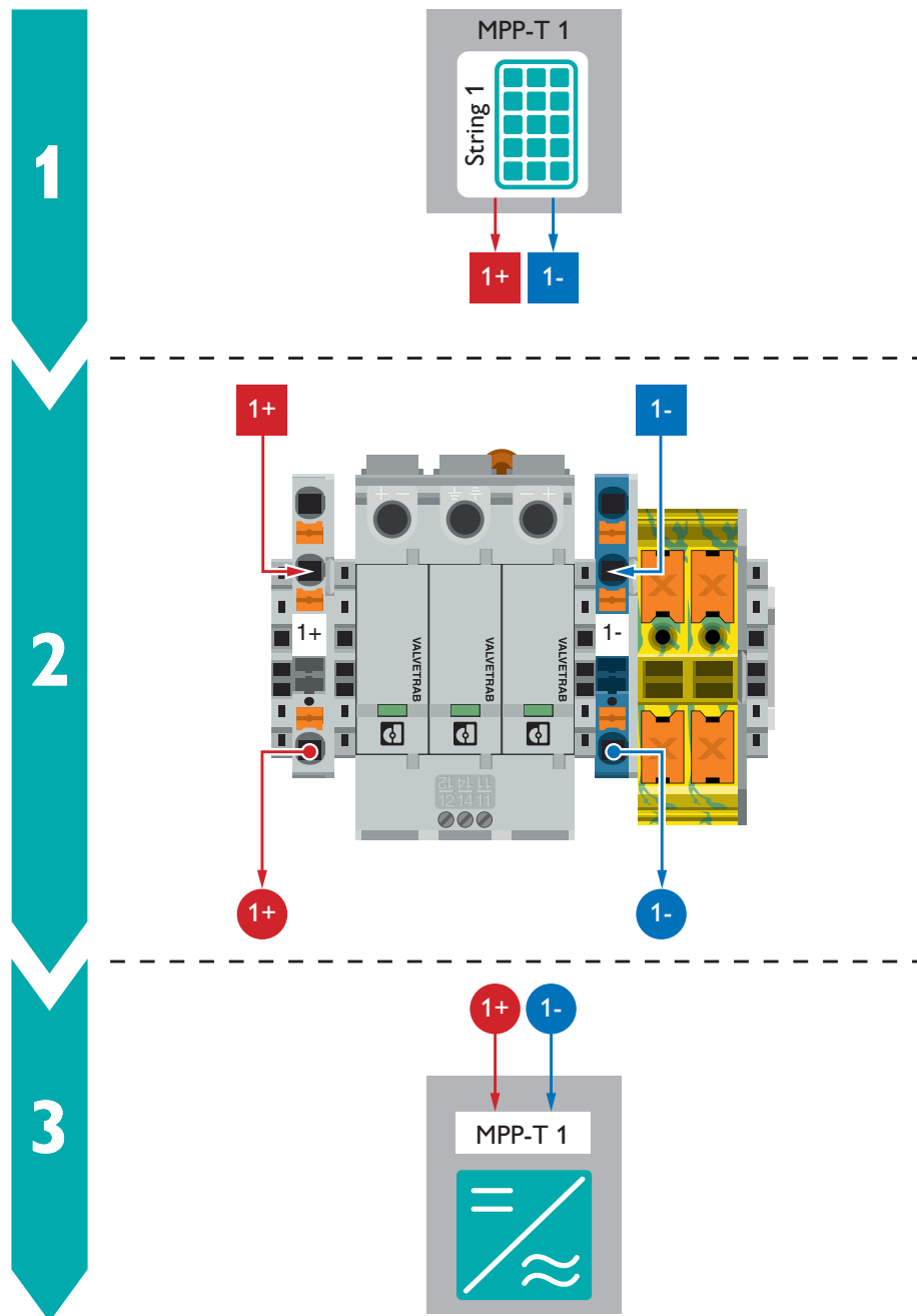
Anschlusszeichnung
