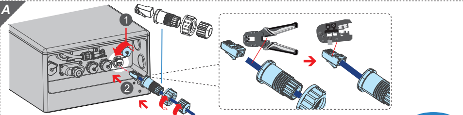
Wechselrichterkabel - RJ45
