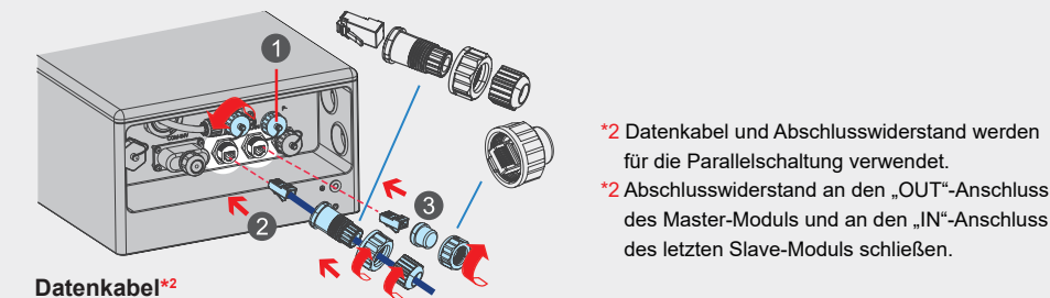
Datenkabel*2
