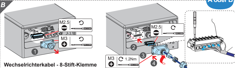
Wechselrichterkabel - 8-Stift-Klemme
